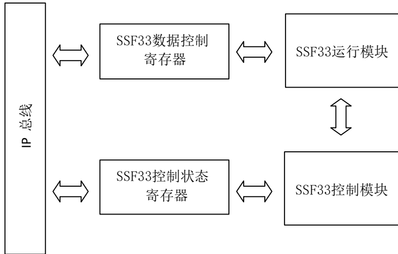
SSF33 算法框架图
